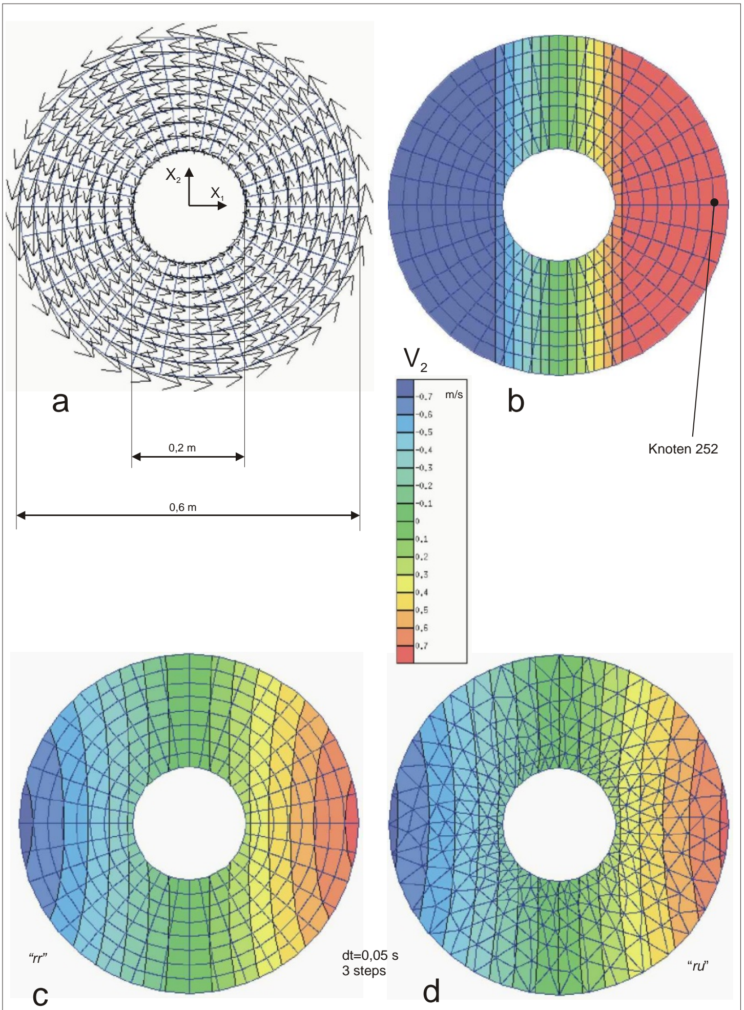
Bild 24. Testfall Starrkörperrotation, a Anfangsbedingung Geschwindigkeitsverteilung, b Anfangsbedingung Isotachen v_2 , c Isotachen v_2 nach 3 s Rechenzeit, regelmäßiges Netz, d dito, unregelmäßiges Netz
