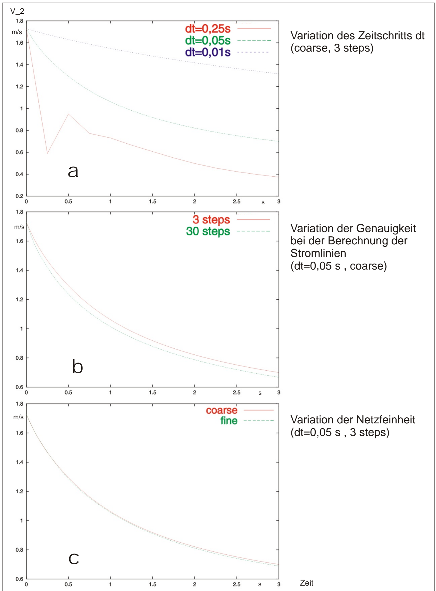
Bild 25. Testfall Starrkörperrotation, numerisch bedingte Geschwindigkeitsabnahme am Knoten 252 (siehe Bild 24b ), a Variation des Zeitschritts dt , b Variation der Genauigkeit in der Stromlinienberechnung, c Variation der Netzfeinheit
