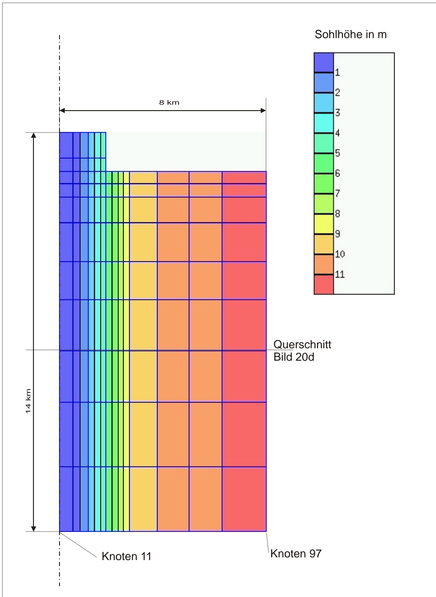
Bild 18. Testfall Tide in einer Bucht, Netz und Topographie
