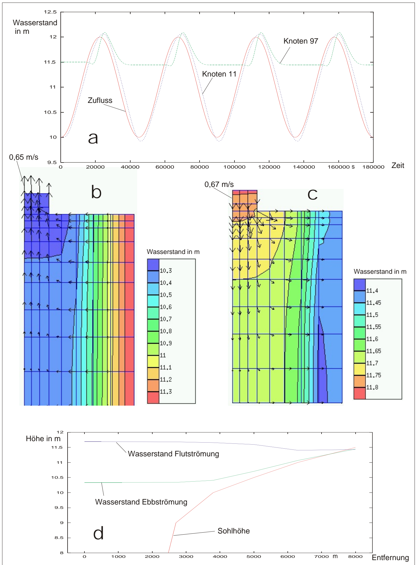
Bild 20. Testfall Tide in einer Bucht, a Wasserstandsganglinien, b Ebb-Strömung 130 500 s = 36,25 h, c Flut-Strömung 153 000 s = 42,5 h, d Querschnitt
