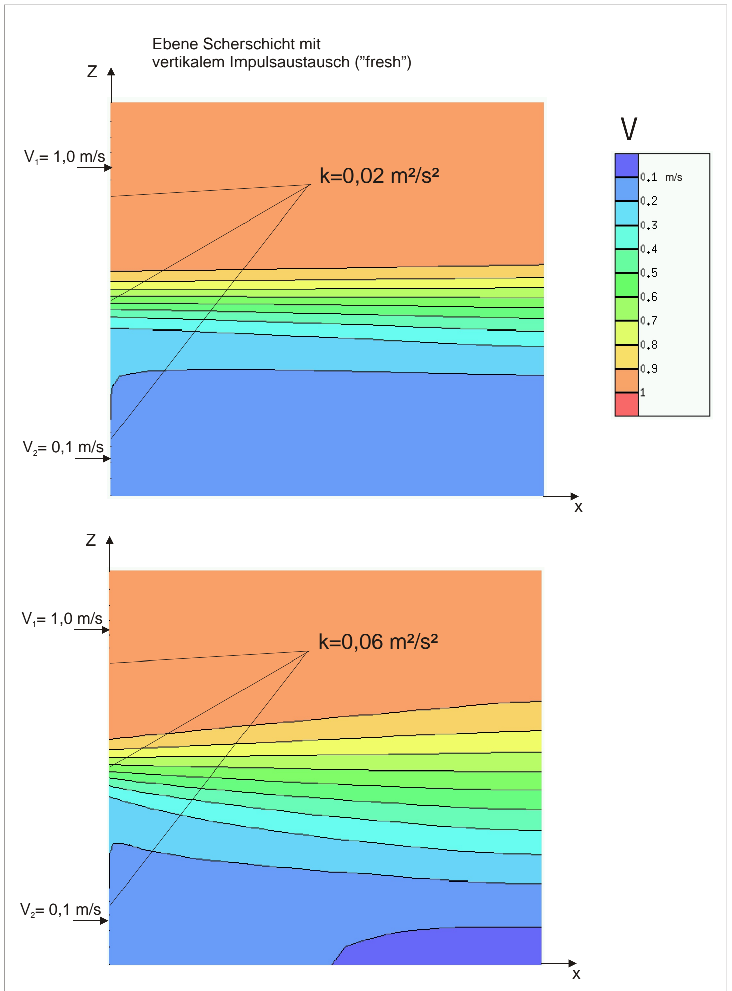
Bild 33. Testfall Ebene Scherschicht, Vergleich unterschiedlicher Zufluss-Randbedingungen für die Turbulenzgrößen
